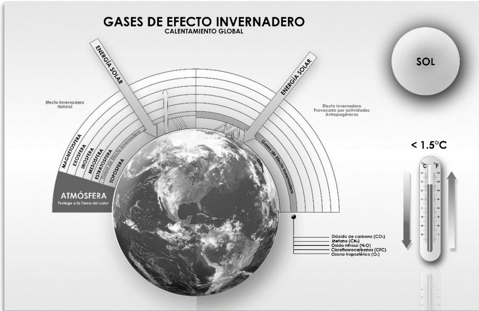
Figura III.3: Descripción del efecto invernadero.
