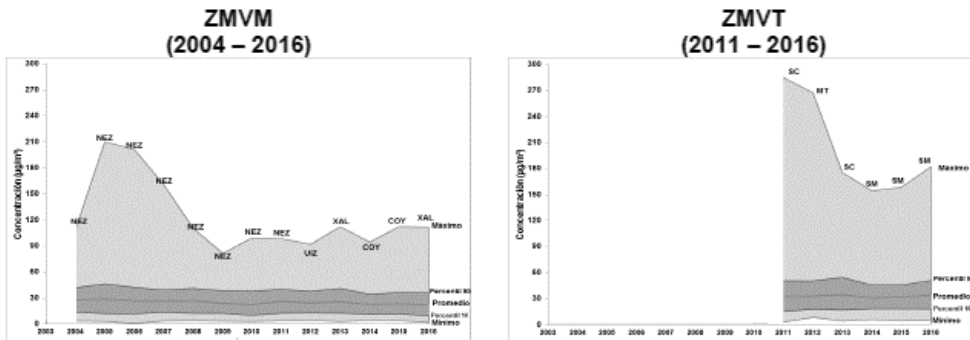
Gráfica IV.18: Tendencia diaria de PM_{2.5} .
