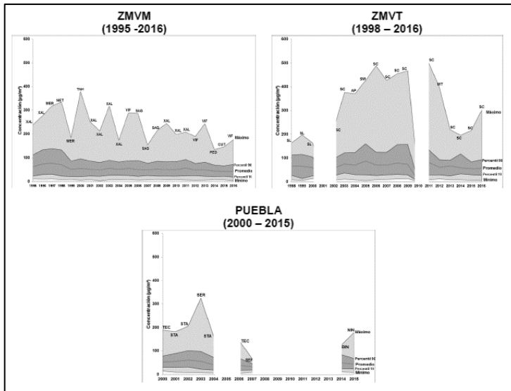
Gráfica IV.17: Tendencia diaria de PM 10 .
