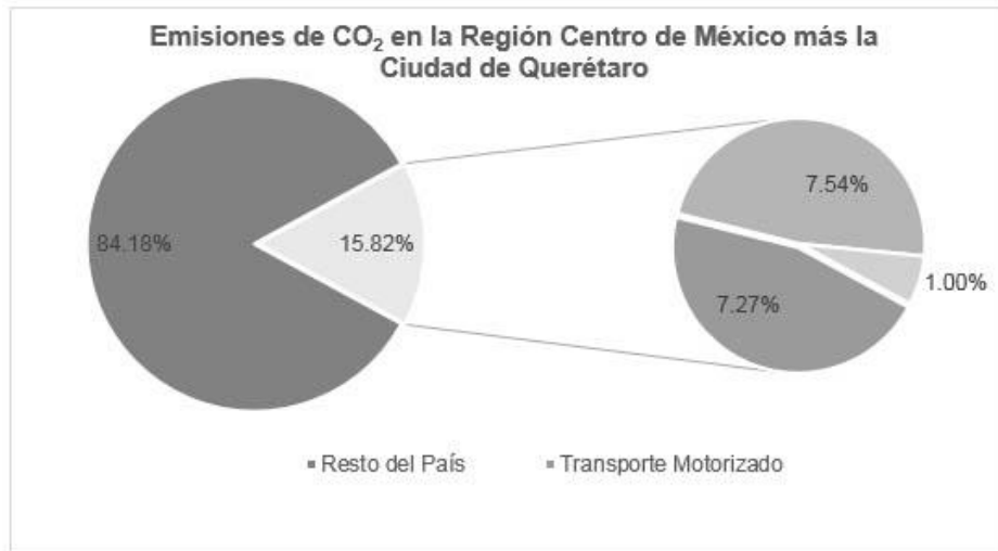
Gráfica III.12: Emisiones de CO 2 en la Región Centro de México más la ciudad de Querétaro.
